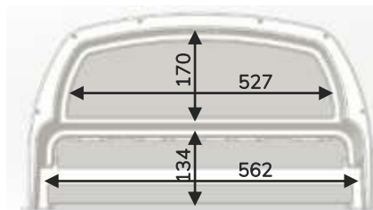
STANDARD DOOR
